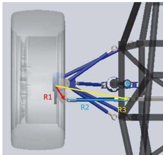
Figura 6. Posicionamiento de los vectores en el ensamble.
